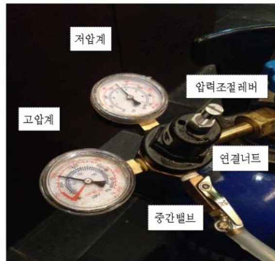
[그림 2-5] 생맥주 압력계
